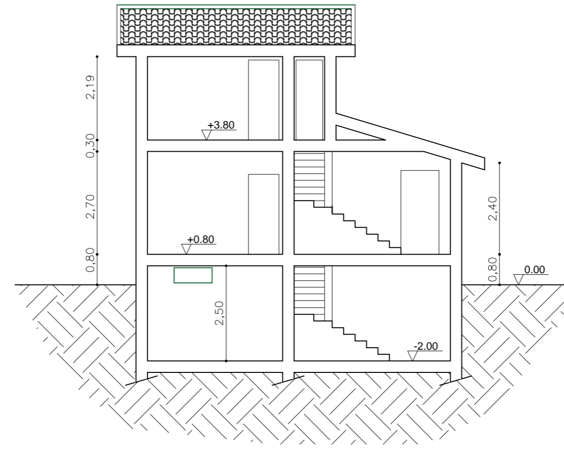
SEZIONE B-B
