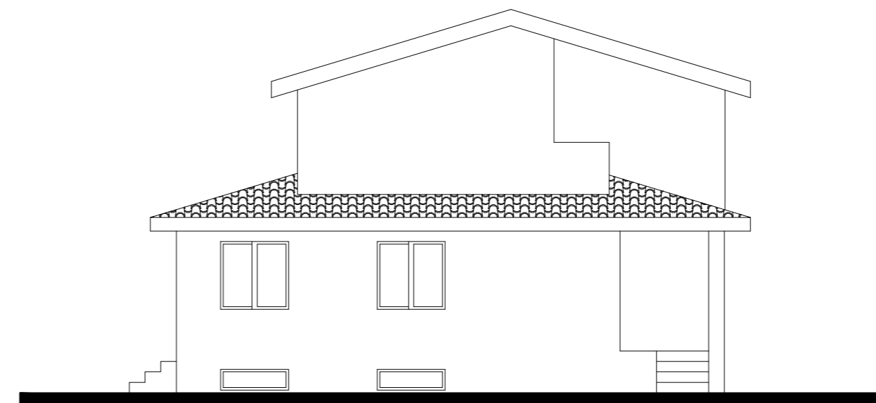
PROSPETTO ANTERIORE
