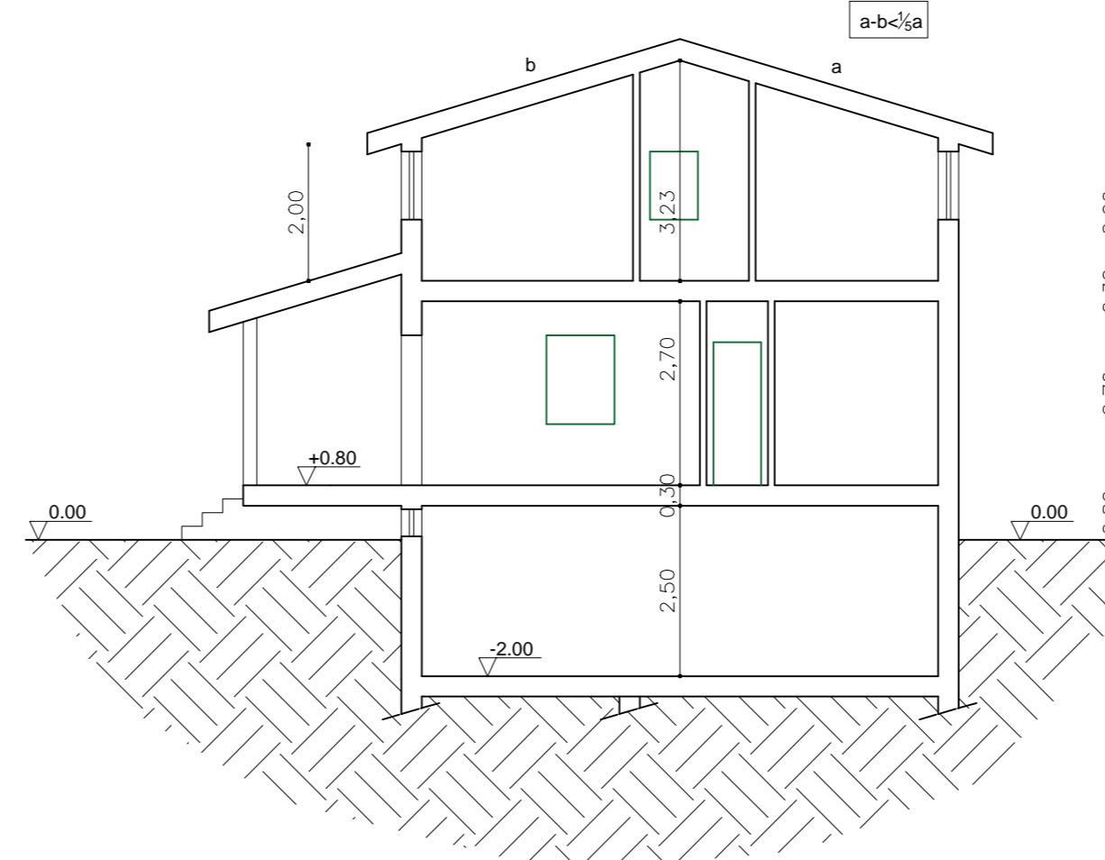
SEZIONE B-B
